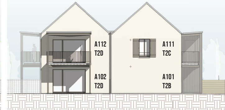
ÉLÉVATION OUEST
